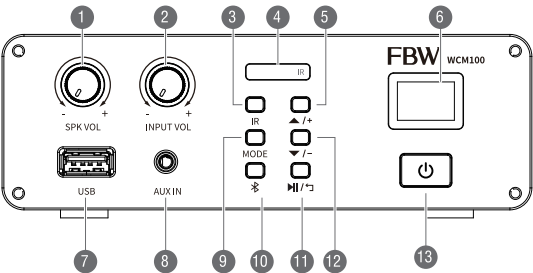
前面板
