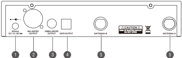
2.后面板
