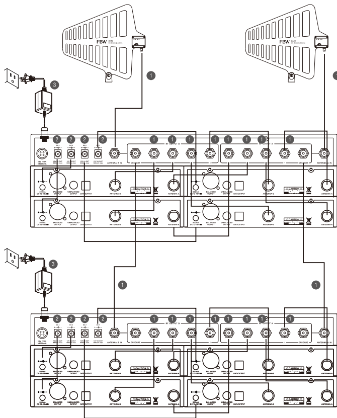
DA40单指向天线与AD82天线分配器连接
